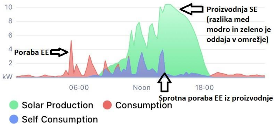
Slika 6: Dnevni prikaz spremljanja porabe in proizvodnje električne energije
